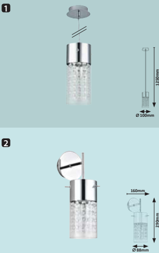
1 6446 GC MG E-14 / 1x max. 40W IP20 • • 19169 chrome/crystal
